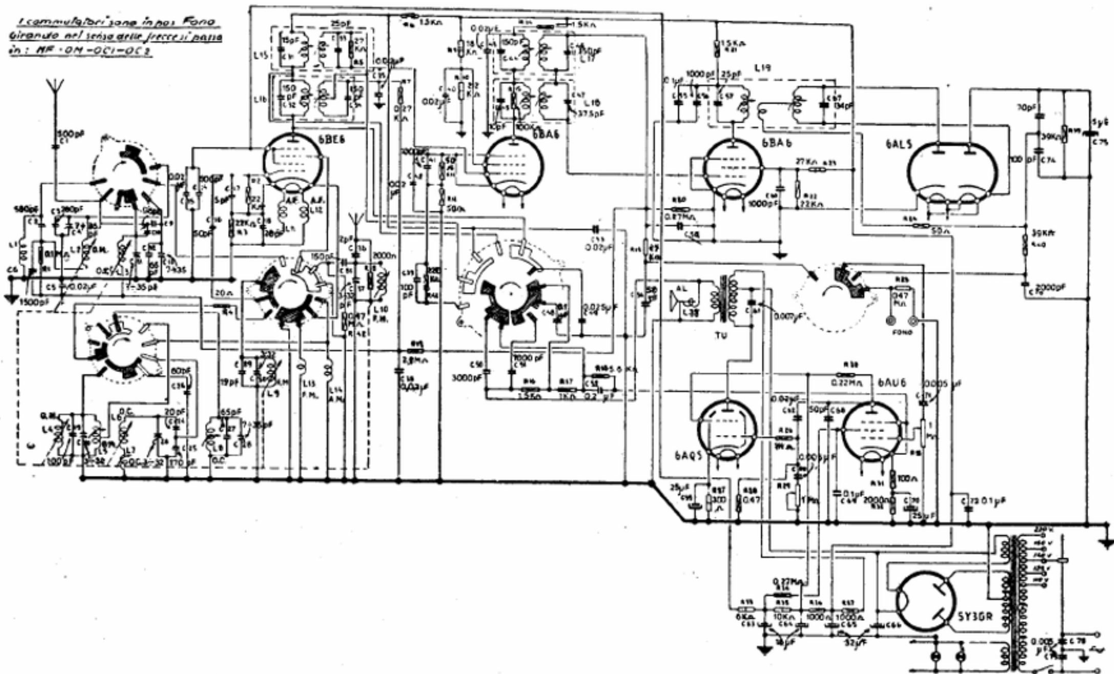
COMPAGNIA GENERALE DI ELETTRICITÀ - Modd. CGE 5107 AM/FM e CGE 6107 AM/FM - Lo schema è del mod. CGE 5107 AM/FM, il mod. CGE 6107 AM/FM è diverso solo per avere l'occhio magico. I commutatori sono in posizione fono. Media frequenza per AM 468 kc; media frequenza per FM 10,5 Mc.
